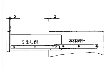
■ レール取付け側面図
