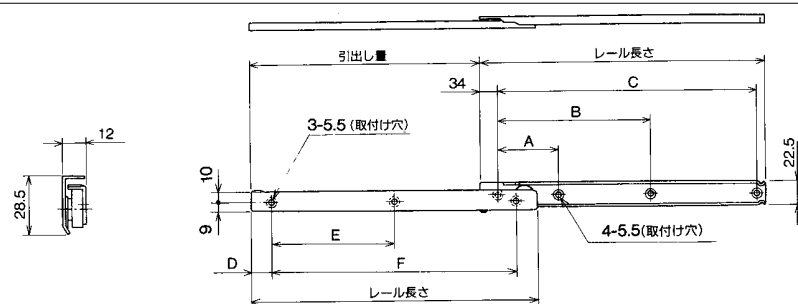
■ レール取付け正面図
