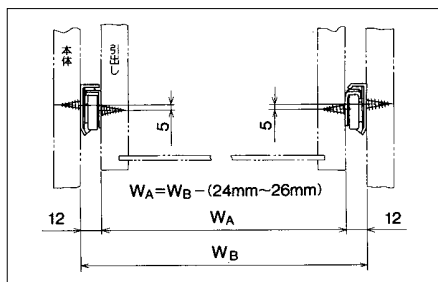
■ レール取付け正面図
