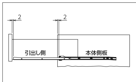
■ レール取付け側面図
