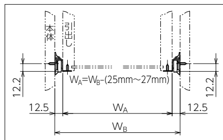
■ レール取付け正面図
