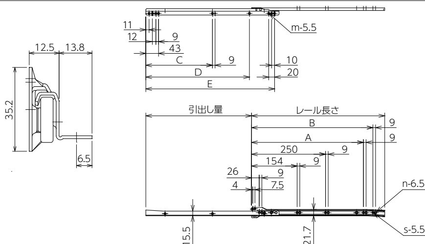
■ レール取付け正面図
