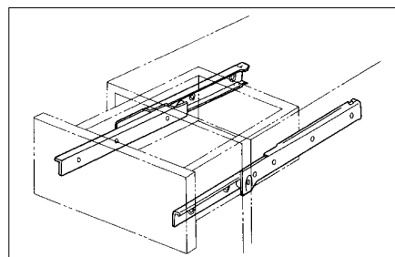
■取付け図
