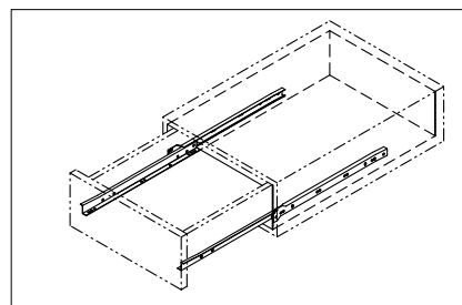
■取付け図
