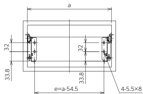
裏板取付け寸法
