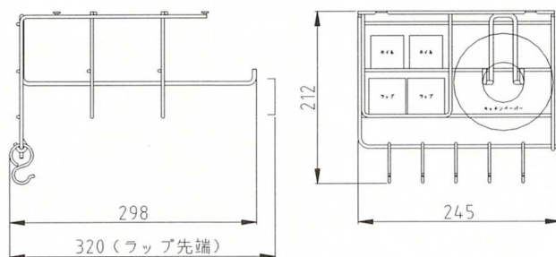
製品寸法
