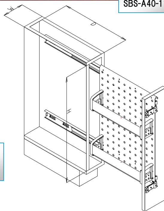
W150 タイプ 写真のモデルは SBS-A40-115
