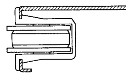
図-3 差込んだ状態断面
