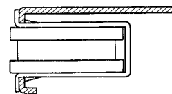
図-3 差込んだ状態断面
